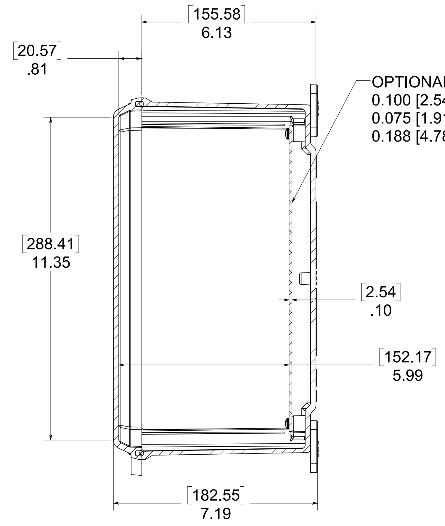
SECTION A-A
