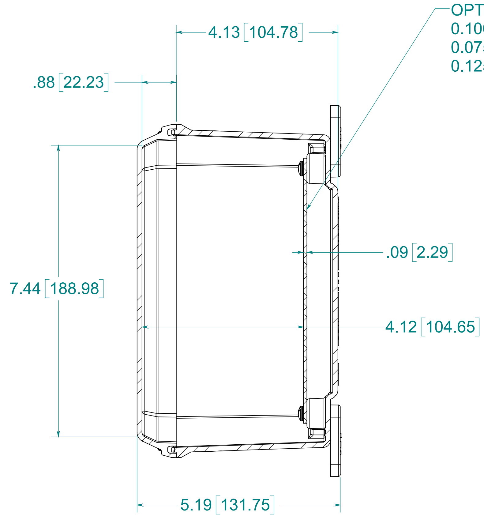
SECTION A-A
